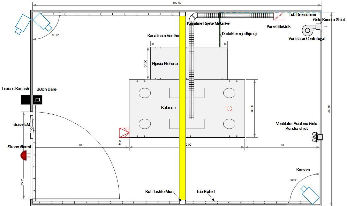
Figura1 - Planimetria e DhomesdhePlanvendosja e Paisjeve
